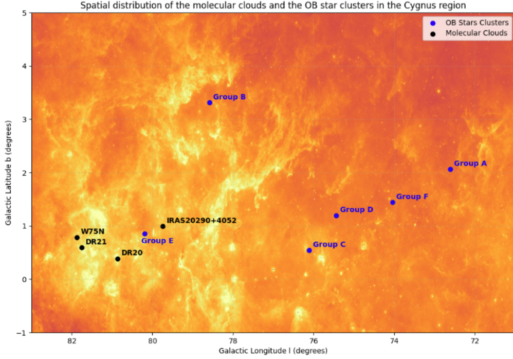
FIGURE 4 – Projection des positions des nuages moléculaires et des groupes d'étoiles massives sur une image WISE à 12 \mu\text{m} . L'abscisse est la longitude galactique et l'ordonnée est la latitude galactique. Les nuages moléculaires sont en noir et les groupes d'étoiles en bleu
